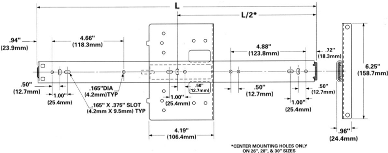
Dimensions
