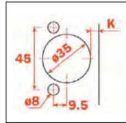
Standard Door Drilling Salice/Blum Pattern
