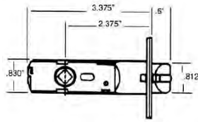
2-3/8" Backset
